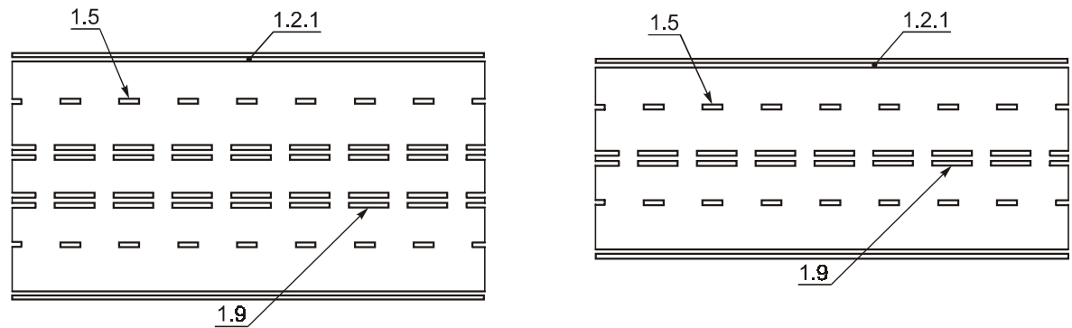
Рисунок В.16 — Примеры нанесения разметки 1.9
