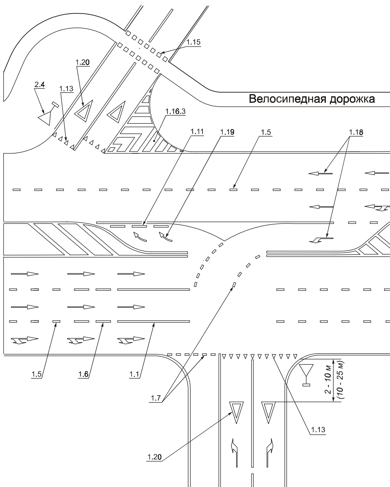
Рисунок В.10 — Пример нанесения разметки канализированного пересечения
