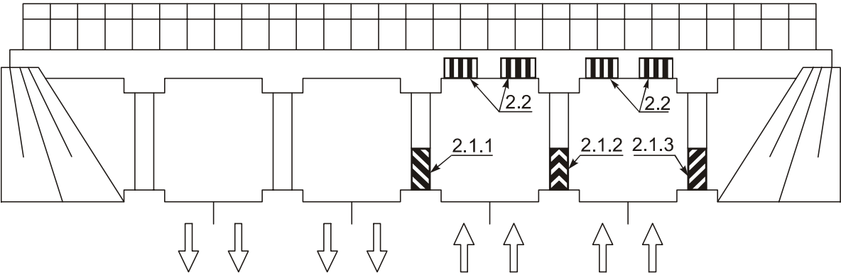
Рисунок В.20 — Пример нанесения разметки 2.1 и 2.2
